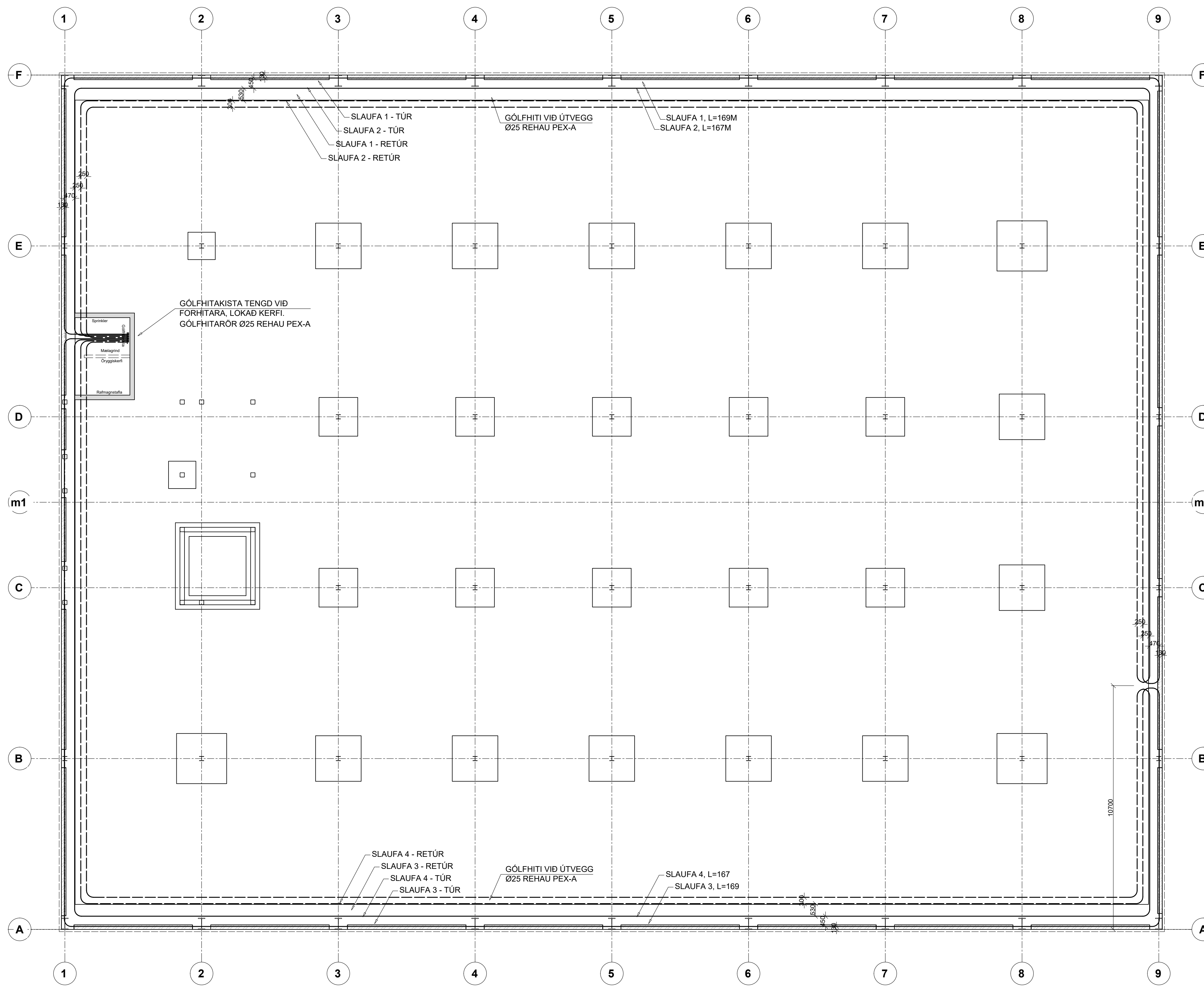
GRUNNMYND, GÓLFHITI 1:100
